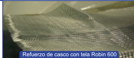
Refuerzo de casco con tela Robin 600
